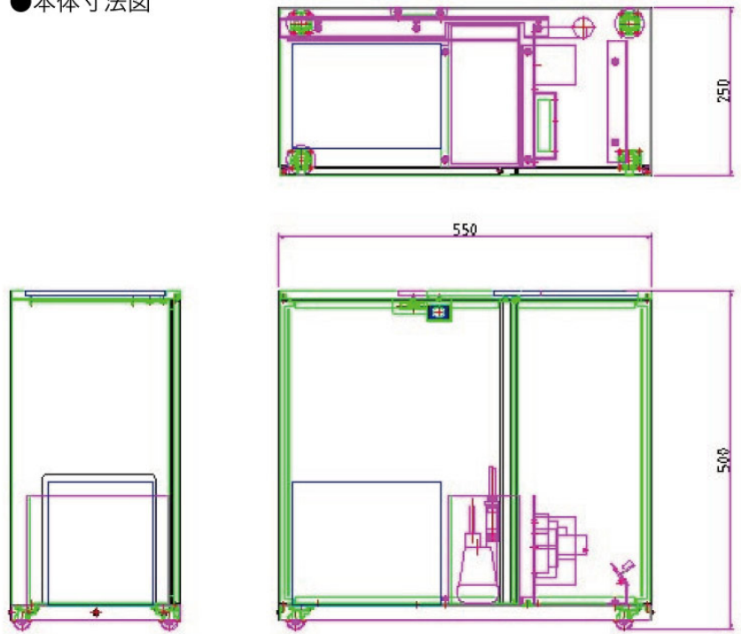
●本体寸法図
